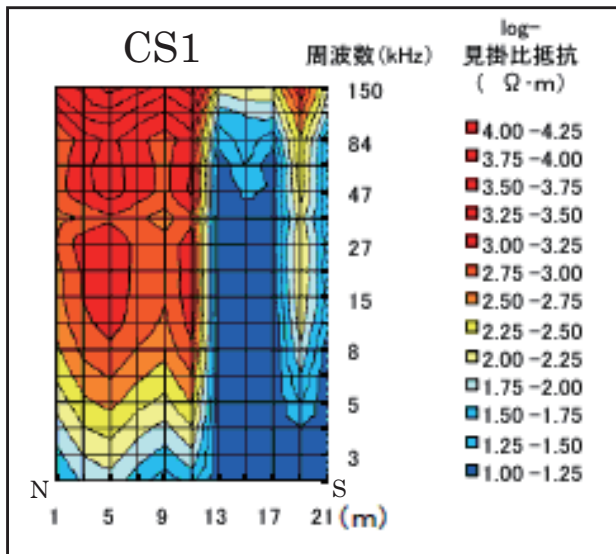
図7 高周波CSMT探索における、CS1測線での見掛け比抵抗の疑似断面図。青色ほど低比抵抗（対数で表示）となる
