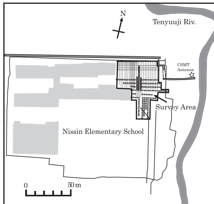
図2 築地反射炉跡があるとされる日新小学校の校舎配置及び調査域、やや濃い部分は水路を示す。細線部は地中レーダ調査域。黒丸は磁気調査測点。星印はCSMT調査用アンテナ設置点
