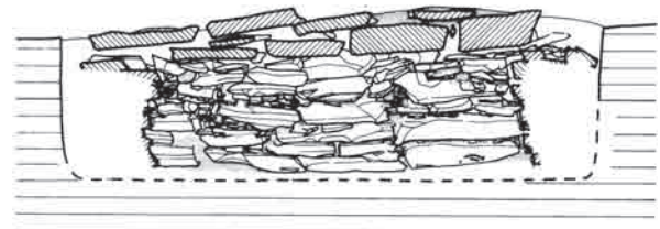
1. 石棺系竪穴式石室1式；佐賀市久保泉丸山 ST006（短壁、長壁とも最下段から板石を小口積み）
