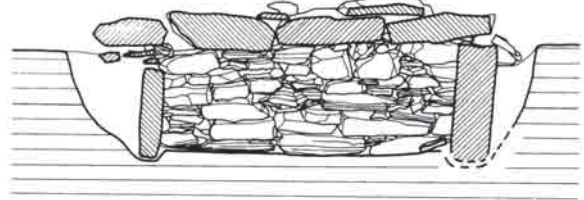
2. 石棺系竪穴式石室2式；佐賀市久保泉丸山 ST007（短壁の最下段にのみ板石を設置）
