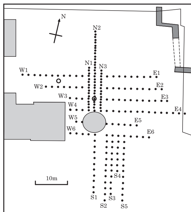
図8 磁気探索測点分布。やや黒い影の部分は水路。丸印は小規模電気探索測点
